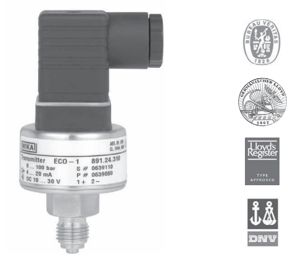
图：ECO-1 型压力变送器适合船用，具有各种国际认证 参见样本 PE 81.18
